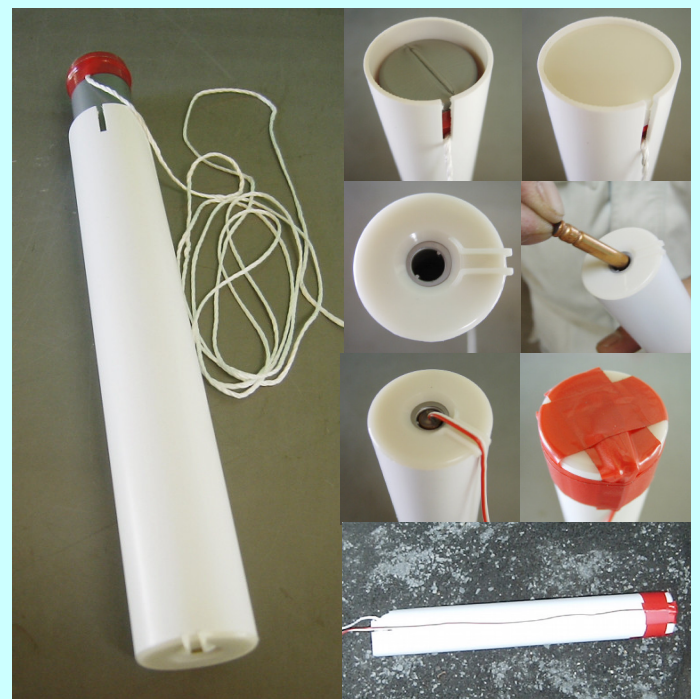
弾性波探査用カートリッジへの挿入と着火具の挿入
